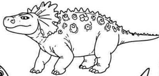
Ankylosaurus
